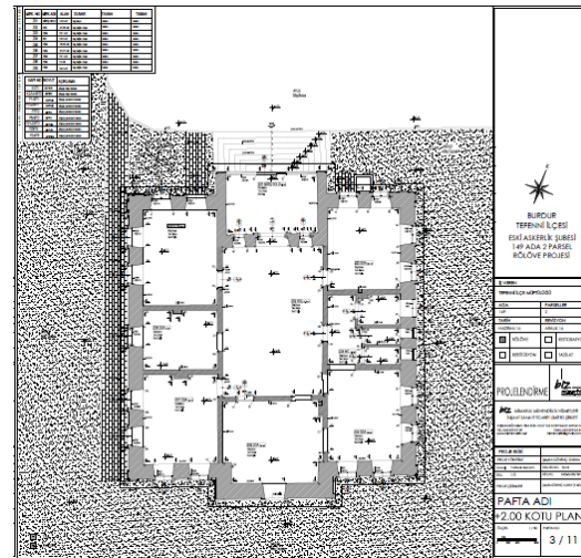
Fig. 2. Tefenni Redif Dairesi Rölövesi Planı (Şeyda Güvenç Duran)
